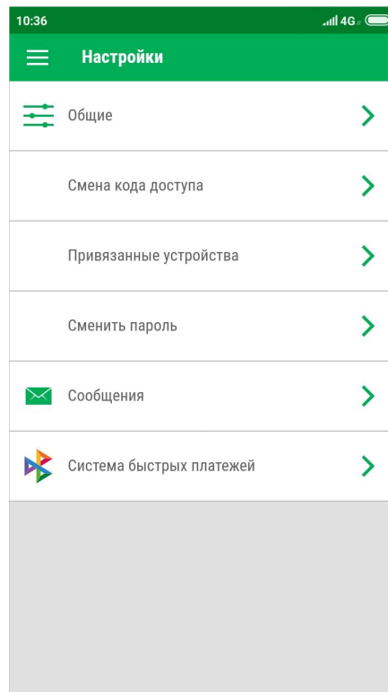
Рис. 25. Раздел "Настройки"
